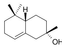
alpha-ambrinol
