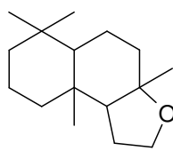
ambrox
